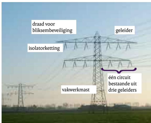
Voorbeeld van een 4-circuits vakwerkmast.
